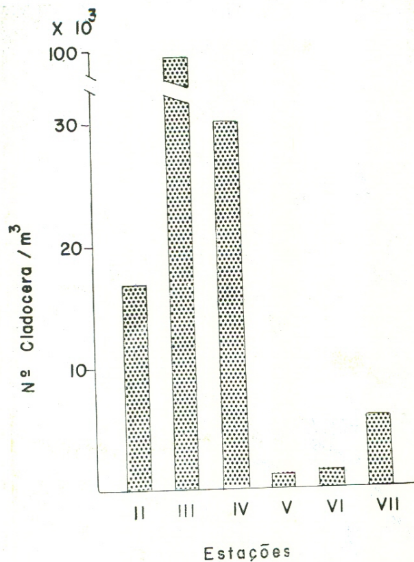
Fig. 8 — "Standing-stock" de Cladóceras na represa de Curuá-Una em abril de 1978.
