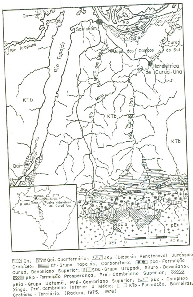
Fig. 1 — Mapa geológico da bacia hidrográfica do rio Curuá-Una.
