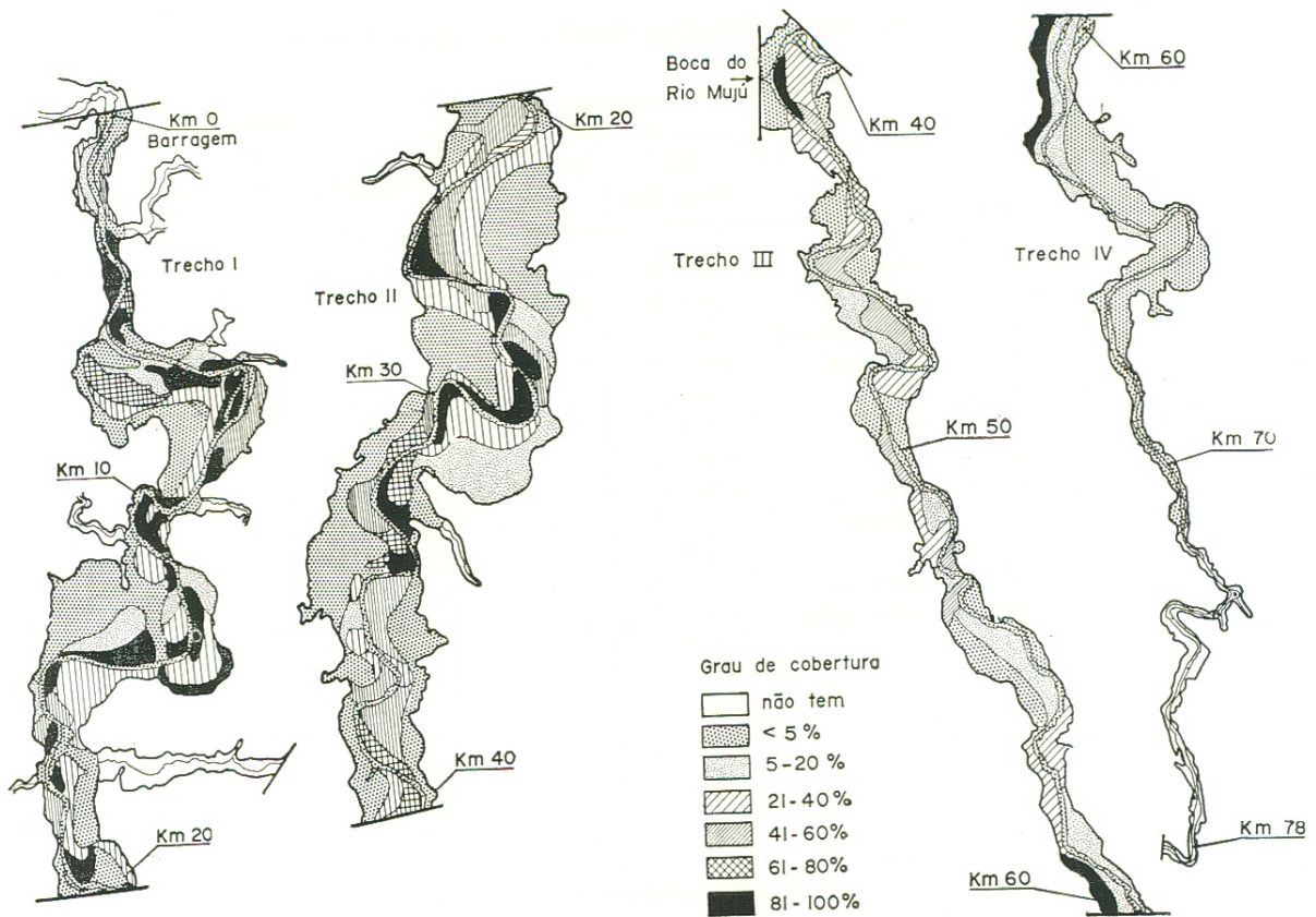
Fig. 5a., b — Grau de cobertura com macrófitas aquáticas nos trechos I e II (Fig. 5a) e III e IV (Fig. 5b) na área influenciada pelo rio Curuá-Una (maio de 1978).
