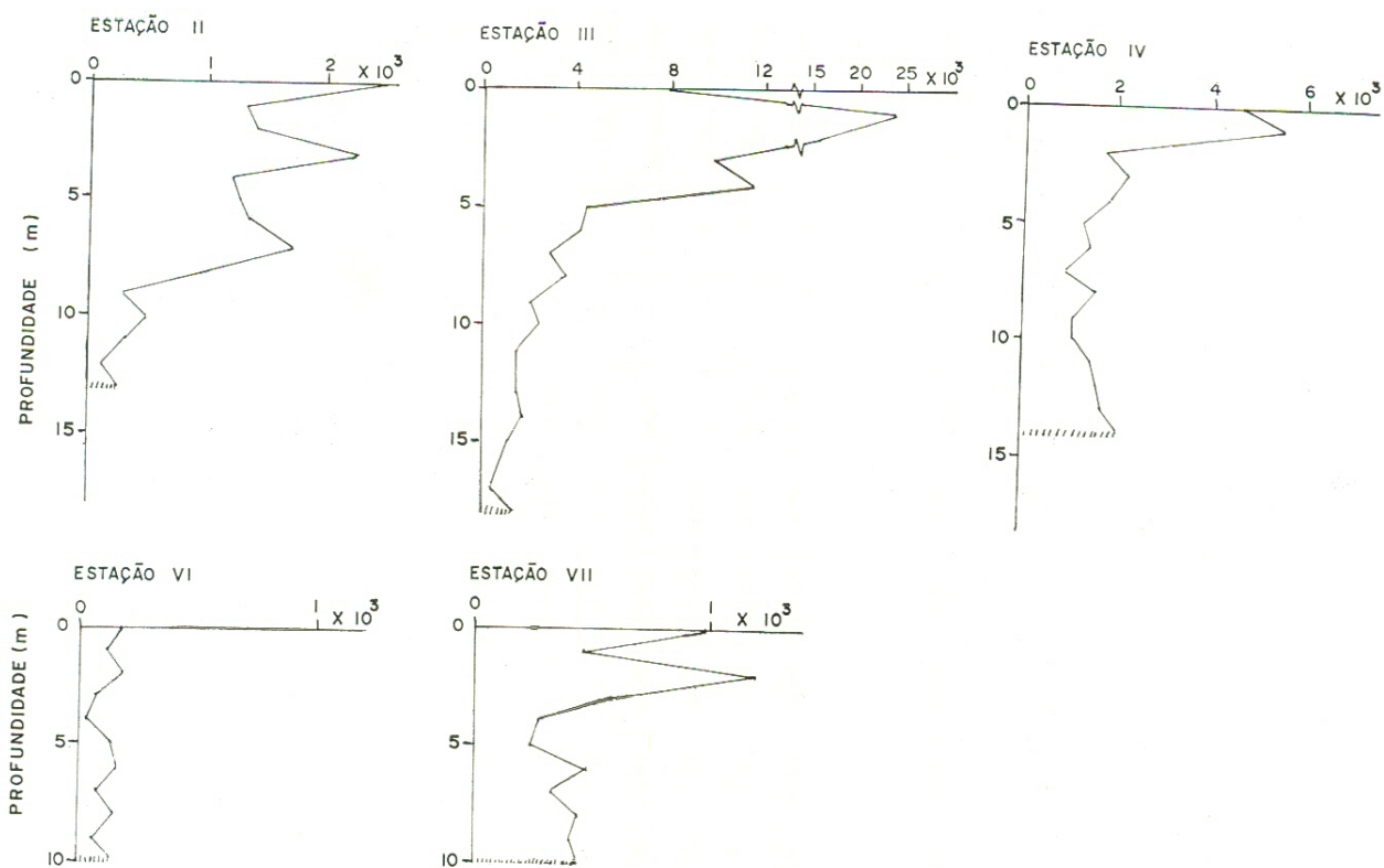
Fig. 9 — Distribuição vertical de Cladóccera (n.º ind/m 3 ) na represa de Curuá-Una em abril de 1978.
