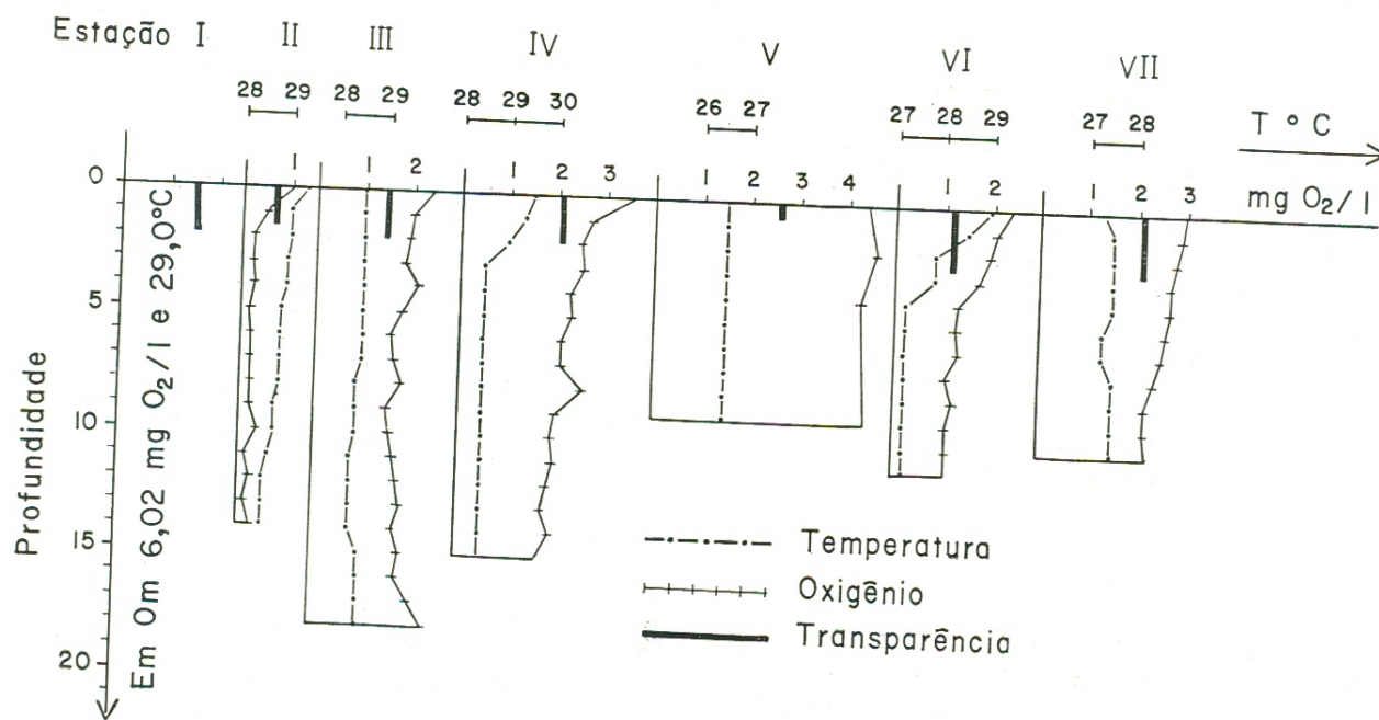
Fig. 4 — Valores de oxigênio, da temperatura e da transparência (profundidade de Secchi) nas diferentes estações da represa de Curuá-Una. (abril de 1978).
