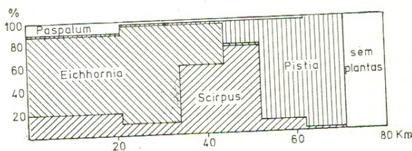
Fig. 6 — Participação percentual das espécies principais de macrófitas aquáticas ao longo do antigo leito do rio Curuá-Una (maio de 1978).
